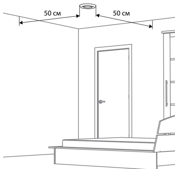
Расположение вытяжной решетки
