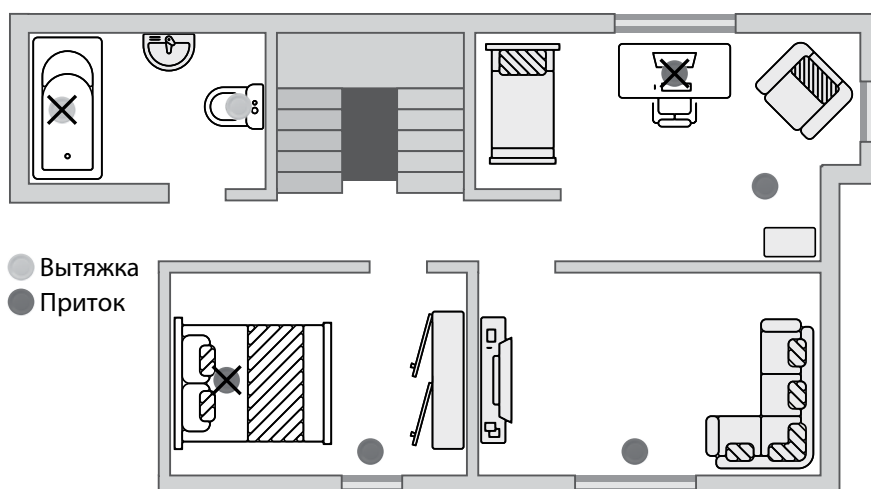
Рекомендации по расположению приточных и вытяжных решеток
