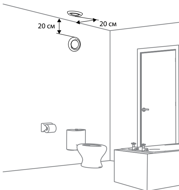
Расположение приточного анемостата
